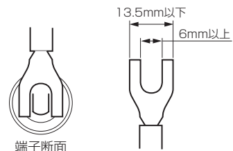
端子断面
