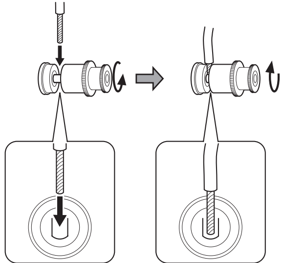
断面図
