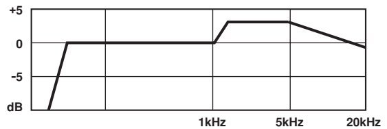
TREBLE ENERGYを「+3」、 TREBLE ROLL OFFを「-2」にセットした場合
