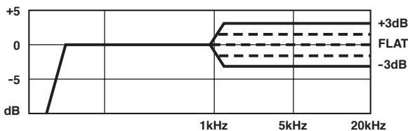
TREBLE ROLL OFFがフラット(LEVELの位置)の場合
