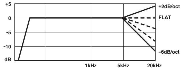
TREBLE ENERGYがフラット(LEVELの位置)の場合
